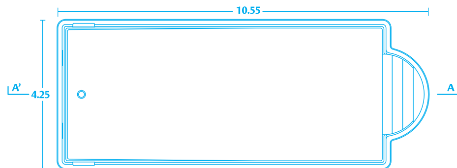
PLANTA / PLAN
