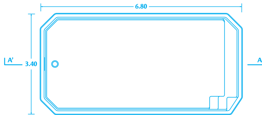
PLANTA / PLAN
