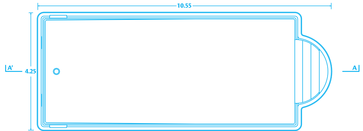
PLANTA / PLAN
