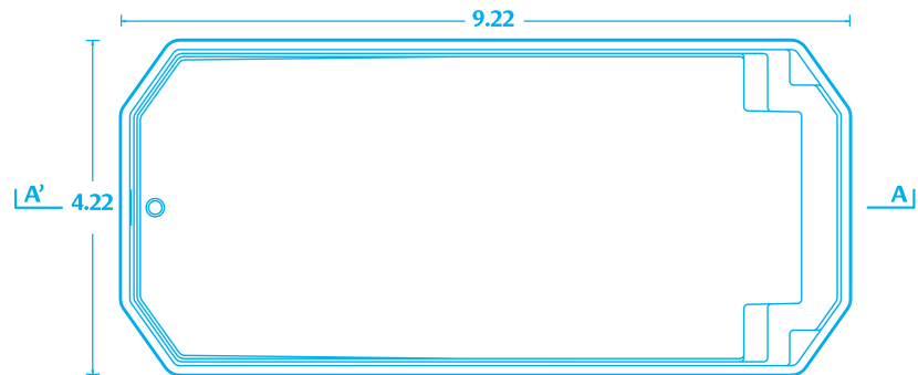
PLANTA / PLAN
