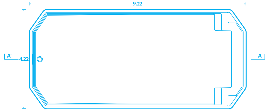
PLANTA / PLAN
