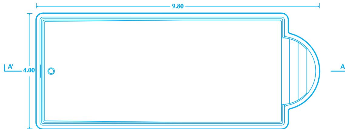
PLANTA / PLAN
